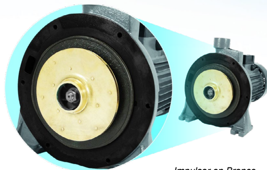
Impulsor en Bronce
